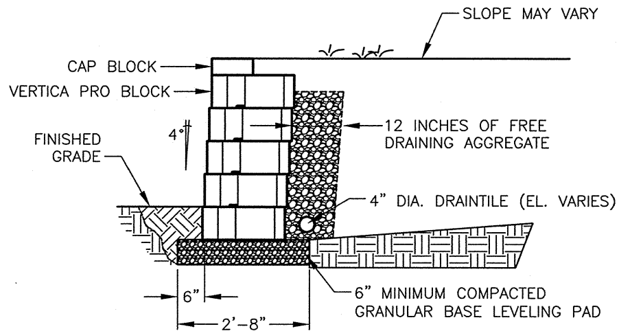
X WX ANCHOR VERTICA PRO® GRAVITY WALL (SCALE: 3/8" = 1'-0")
